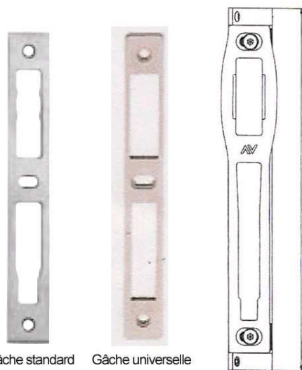
Gâche réglable
