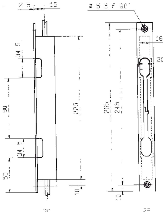
COFFRE À LEVIER N°32
