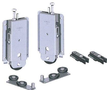
Garniture extérieure
