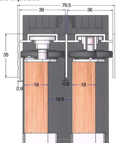
Détail guide haut à roulement + téton et butée loqueteau
