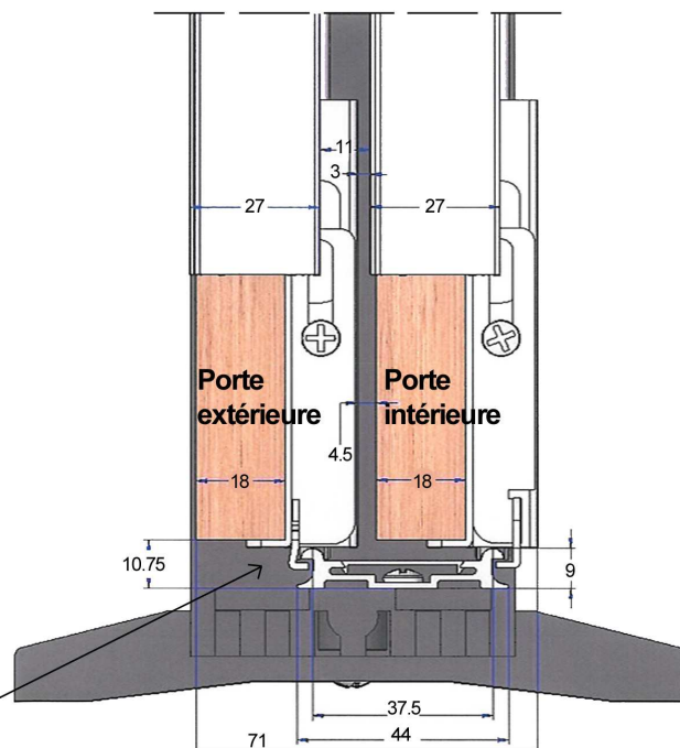
Détail roulement inférieur avec nouveau dispositif anti dégonflage
