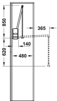
Dispositif d'inclinaison
