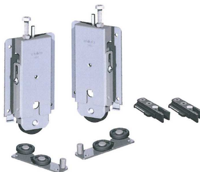
Garniture intérieure
